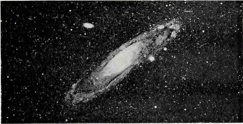
Andromeda-vetrarbrautin.
