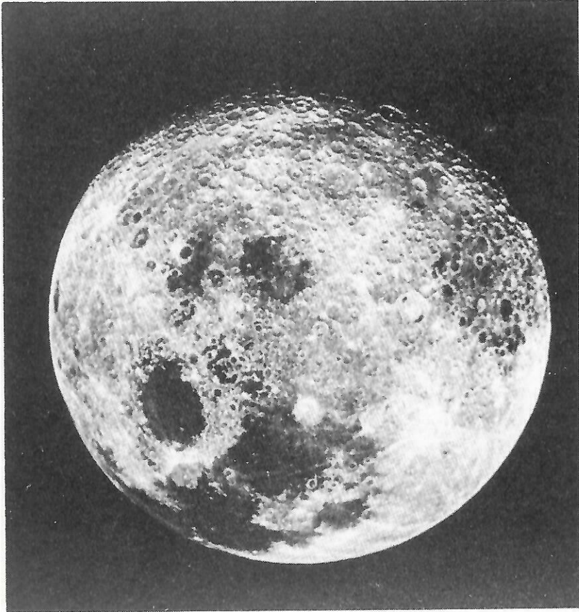
Tunglið, sú hliðin sem að jörðu snýr. (The Hamlyn Guide to Astronomy, bls 168)
