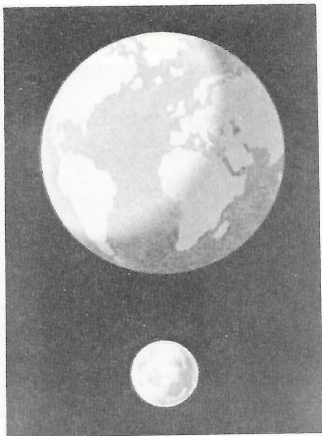
Myndin sýnir stærðarhlutföllin milli jarðar og tungls. (Exploring the Planets bls. 66)
