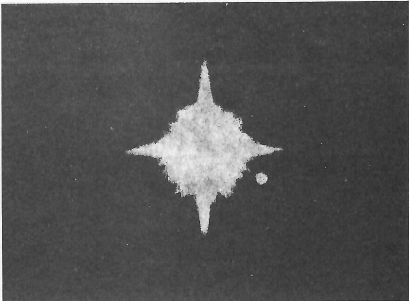
Síríus, hin sindurbjarta, hvíta sól ásamt fylgihnetti hennar.
